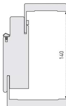
Telaio con coprifilo aletta lunga fino a 140 mm
