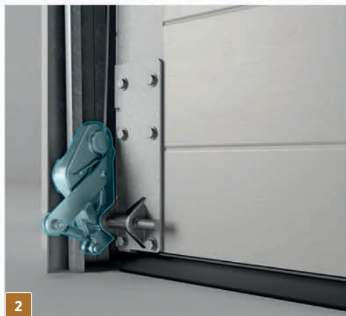
Protezione in caso di rottura della fune - standard nei portoni da garage a due postazioni
